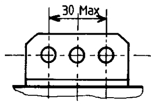
Cadène à trous autorisée
