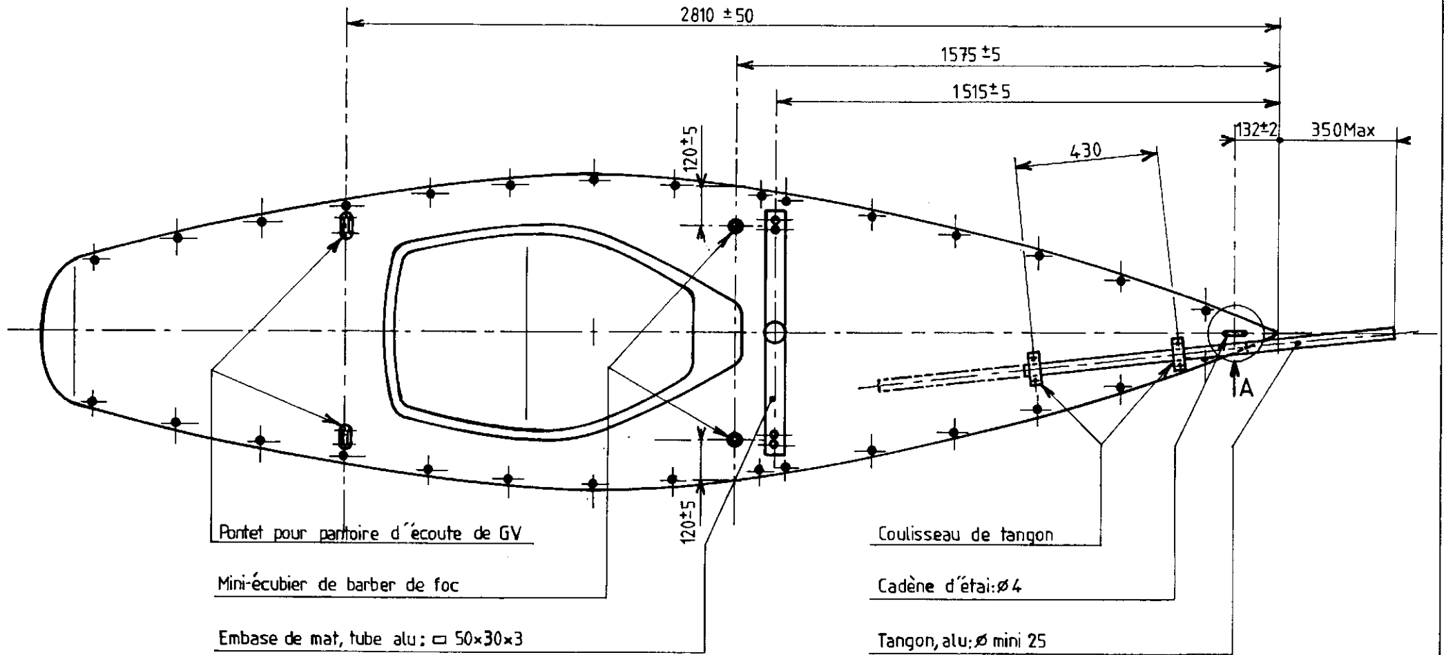
Détail A Echelle: 1:1
